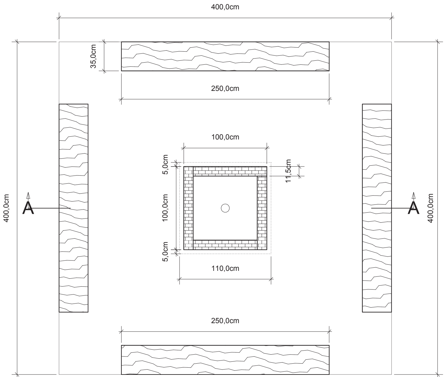
Grundriss 1/20
